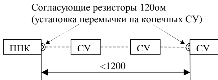
Рис. 4 Подключение сетевых устройств на линию RS-485.
