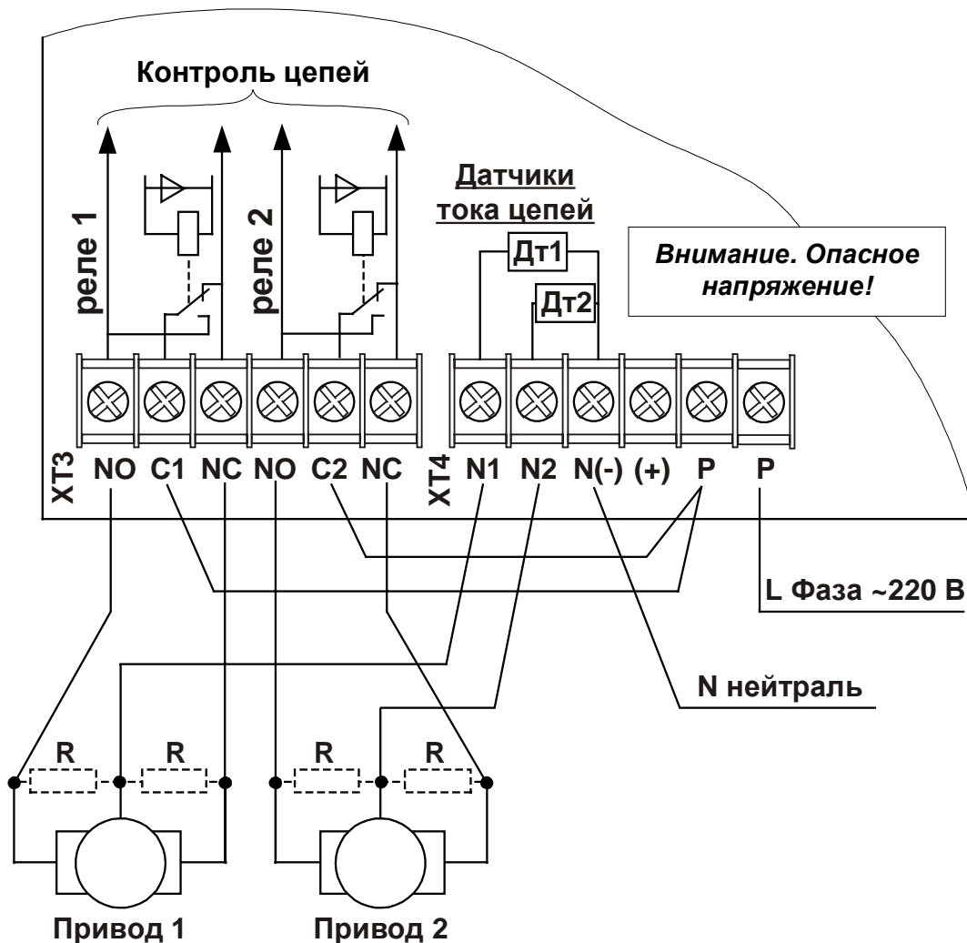
Рис. 5 Подключение 2-х реверсивных приводов переменного тока типа Белимо.
