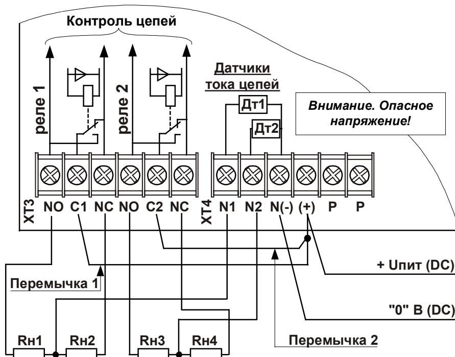
б) Подключение нагрузок к сети постоянного тока =Упит, U_{пит} - (11 \dots 50) В, I_n \leq 3 А
