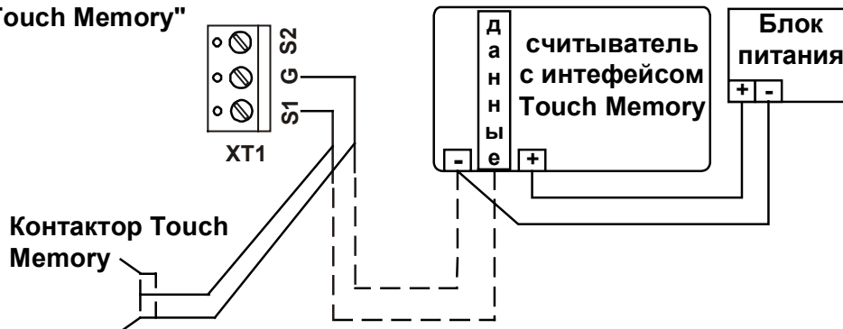
Рис. 10 Подключение контактора или считывателя(пунктиром) Touch Memory
