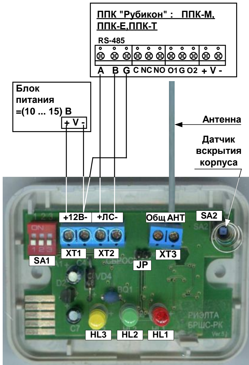
Рис. 2 Расположение элементов, подключение КР.
