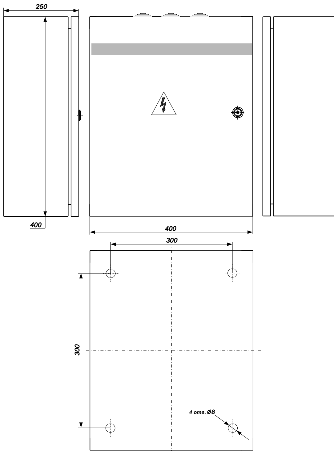
Рисунок 2 – Внешний вид ППК-Р. Габаритные и присоединительные размеры
