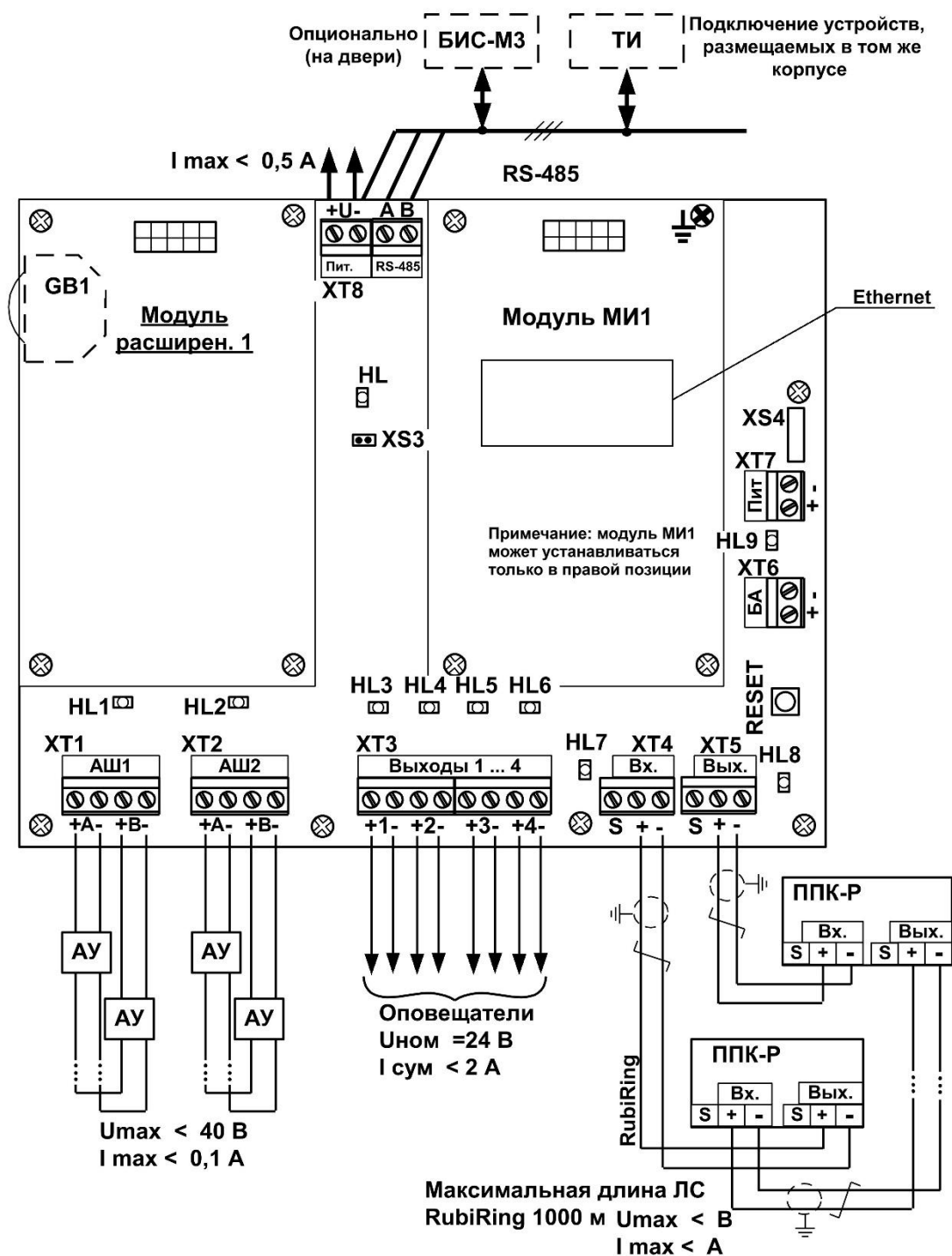
Рисунок 4 – Плата ППК-Р. Подключение внешних цепей
