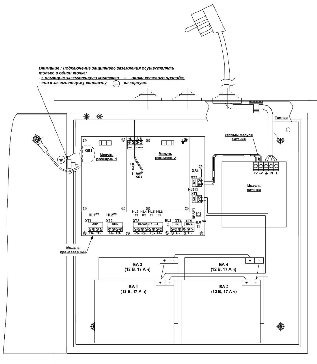
Рисунок 3 – ППК-Р. Расположение элементов. Подключение БА
