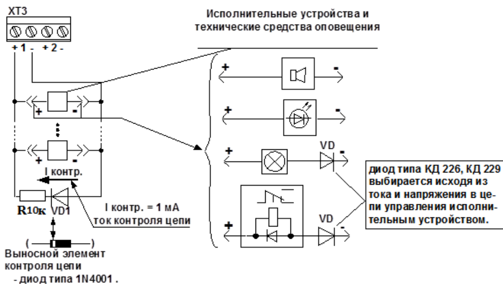
Рисунок 5 – Подключение различных типов ИУ к токовому выходу ППК-Р
