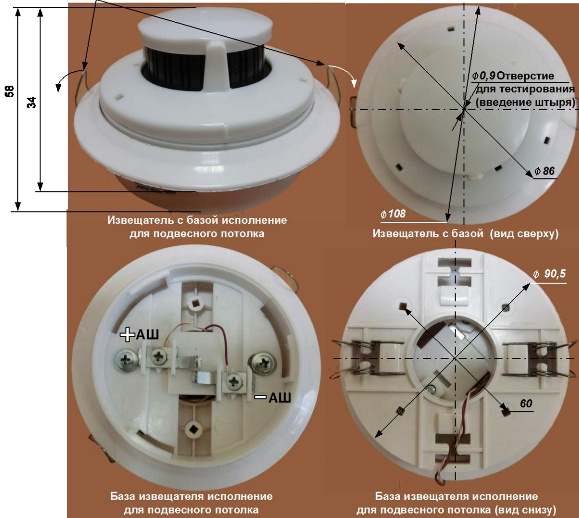
Рис. 4 АЗДПИ. Извещатель с базой для подвесного потолка. Габаритные и присоединительные размеры
