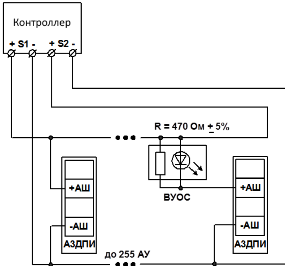
Рис. 5 Подключение АЗДПИ в АШ. Подключение ВУОС.
