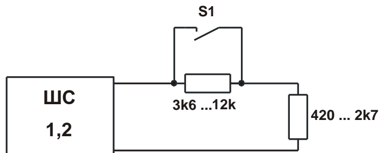
Рис. Схема 4 а) Параллельное подключение одного извещателя с НР контактами. б) Последовательное подключение одного извещателя с НР контактами
