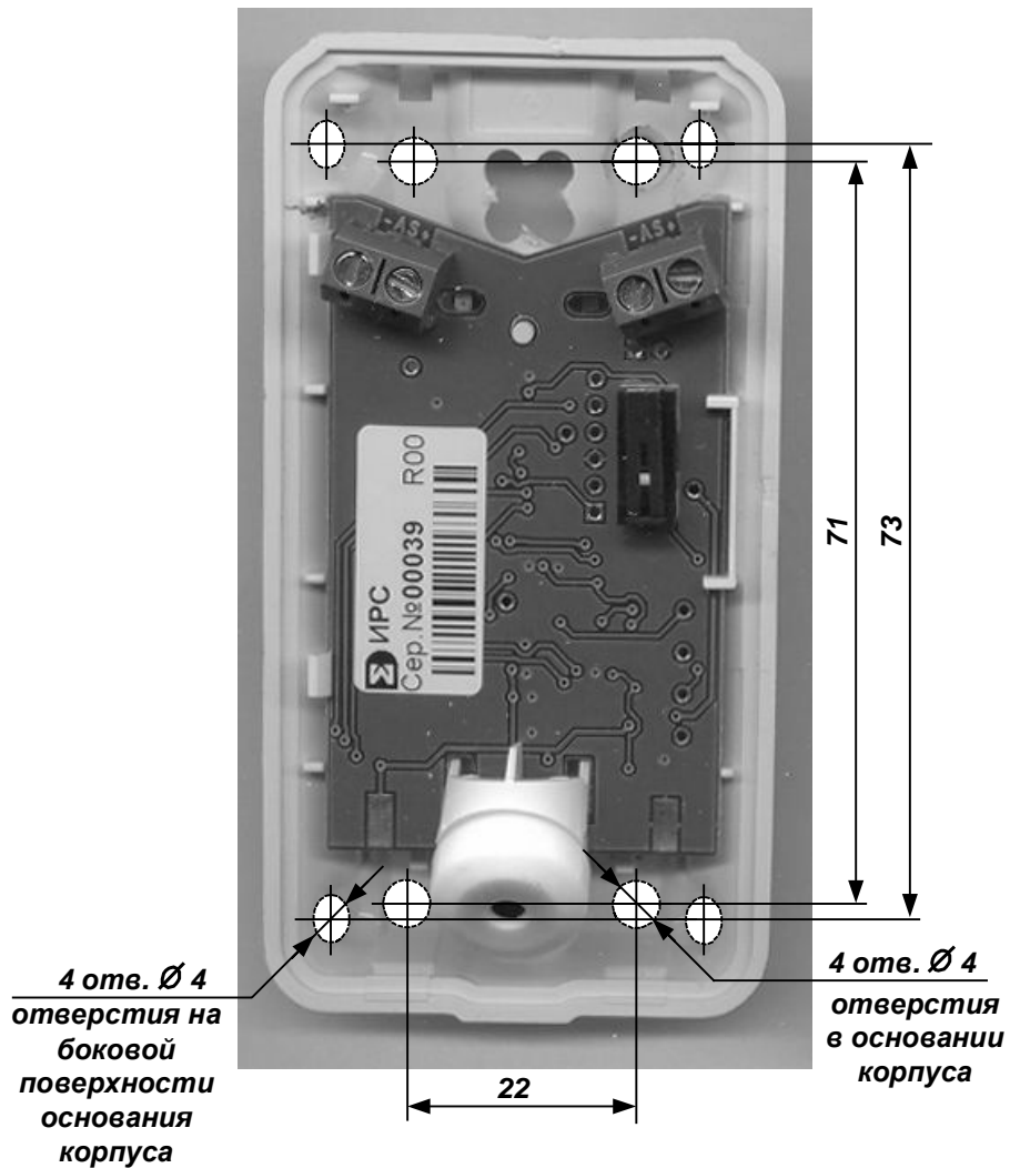
Рис. 3 Присоединительные размеры
