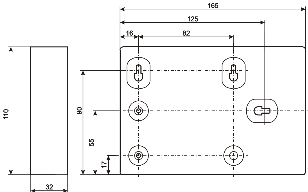
Рис. 2 Габаритные и присоединительные размеры (исполнение IP20)
