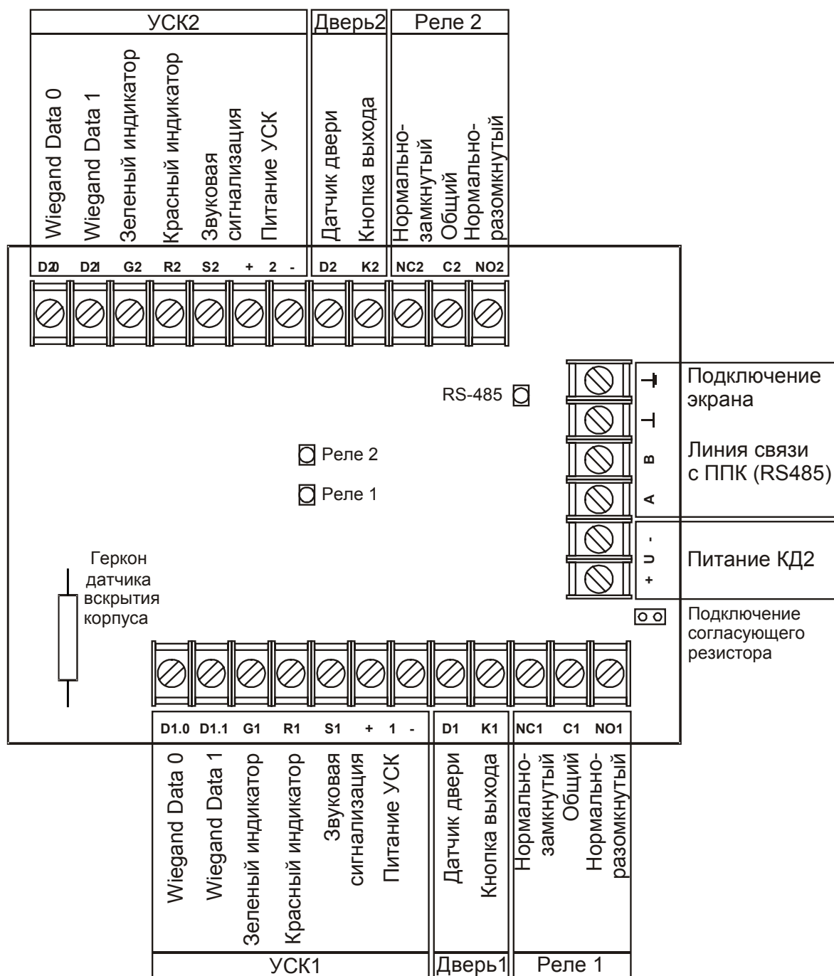
Рис. 5 Клеммы подключения КД2
