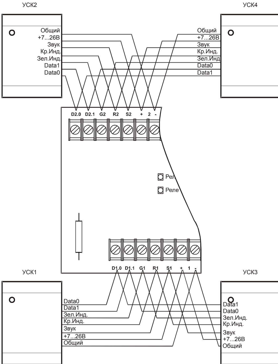
Рис. 6 Подключение УСК для двусторонней ТД
