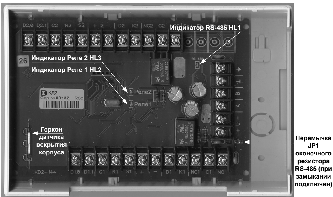
Рис. 1 Внешний вид, расположение элементов
